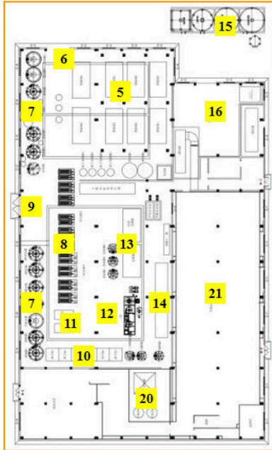
8. Filtration 棉饼过滤工序
