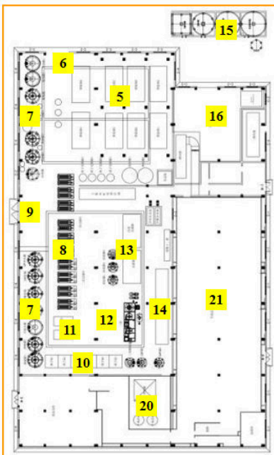
12&13. Evaporation & Sterilizing 蒸发器 & 高温灭菌
