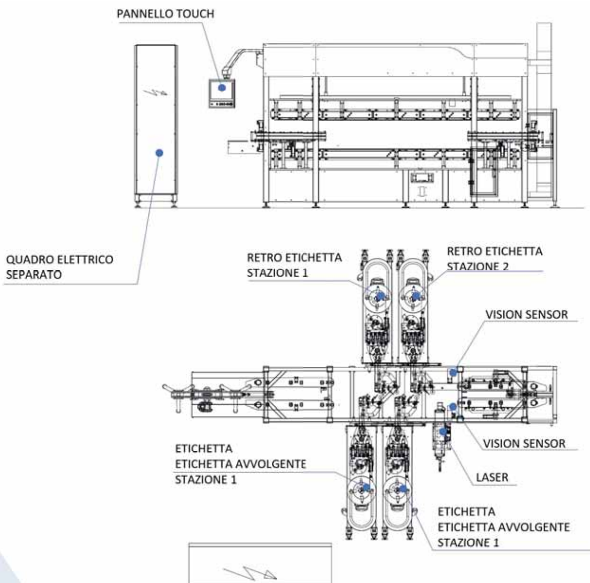
Esempio layout con configurazione macchina con 4 stazioni
