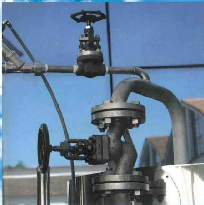
PARTICOLARE SURRISCALDATORE DI VAPORE E VALVOLA DI INTERCETTAZIONE DETAIL OF STEAM OVERHEATER AND ON/OFF VALVE
